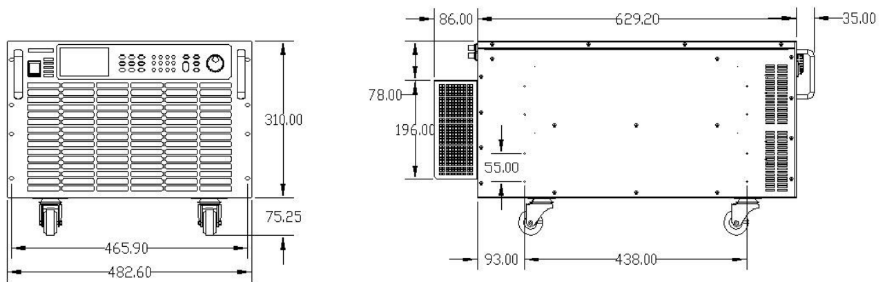
7U机型（8kW~12kW）尺寸图
