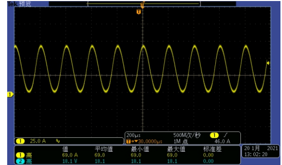
5kHz正弦波
